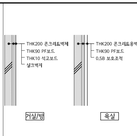
5 | 간접외기벽체상세도
