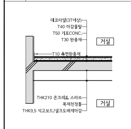
2 표준바닥마감상세도
