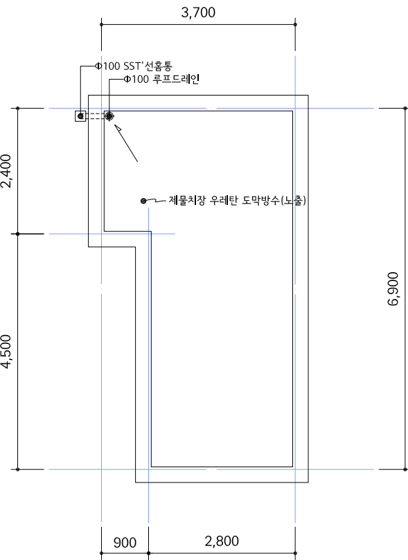
옥탑지붕 평면도 축척 : 1/100
