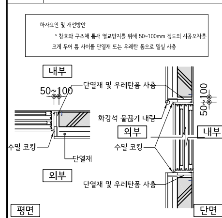
4 창호설치 단면상세도 - 석재마감
