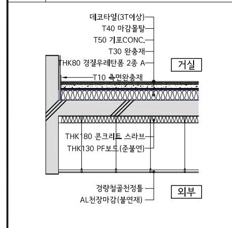
3 | 2층바닥마감상세도
