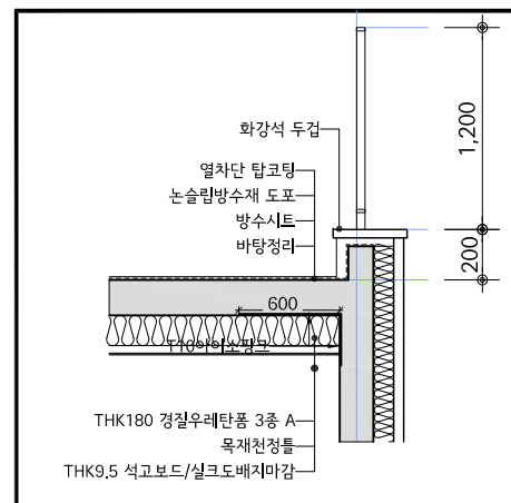
1 파라펫 상세도
